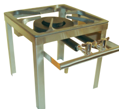
GS11/S 30CM LARG.40CM PROF. 30CM ALT ESTRUTURA EM AÇO INOX GRELHA FERRO FUNDIDO 30X30CM QUEIMADOR DUPLO 15X7CM (opcional com queimador simples 11cm)
